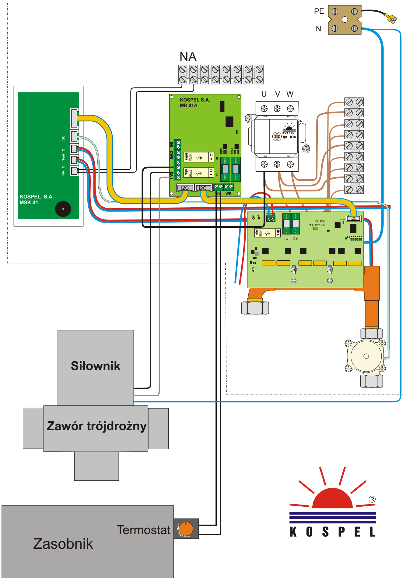
Schemat podłączenia płytki MR 01A, zaworu trójdrożnego i termostatu zasobnika.
