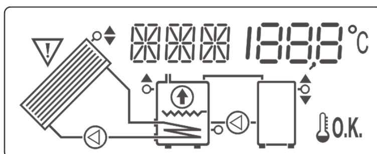
Ilustracja 2: Wyświetlacz ciekłokrystaliczny regulatora Immsol 11
