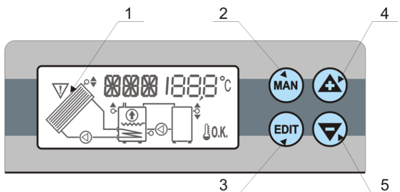
Ilustracja 1: Rozmieszczenie elementów na panelu czołowym
