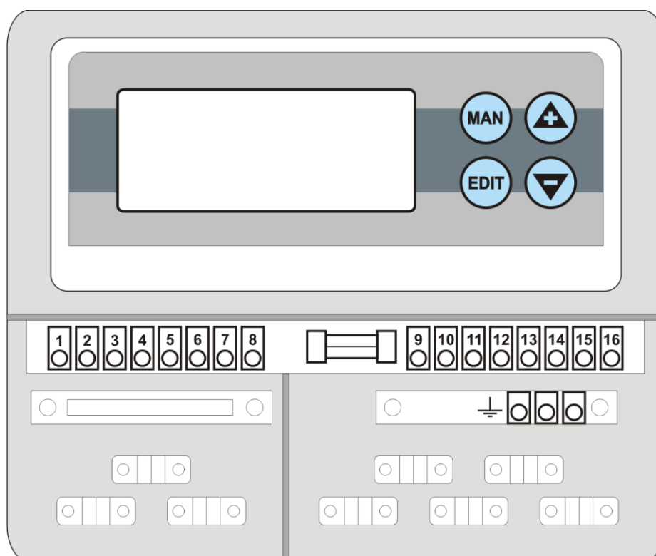
Ilustracja 11: Widok poglądowy regulatora Immsol 11
